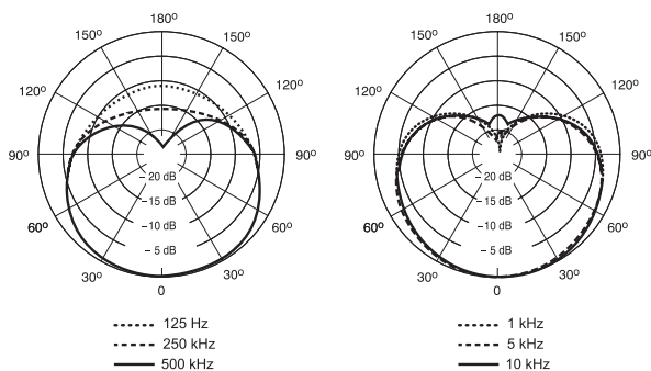
Richtcharakteristik
