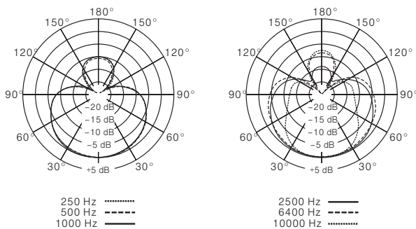
Richtcharakteristik
